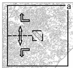
Рис. 3. Подготовка изображения для испытания гидродинамической модели (на примере НТРУ): а – направление разворачивания исходного изображения; б – развернутое изображение; в – карта гидродинамического моделирования, светлым показаны структуры протекания. Заштрихованная часть изображения – выемка. Стрелками показаны направления разворачивания изображения.
